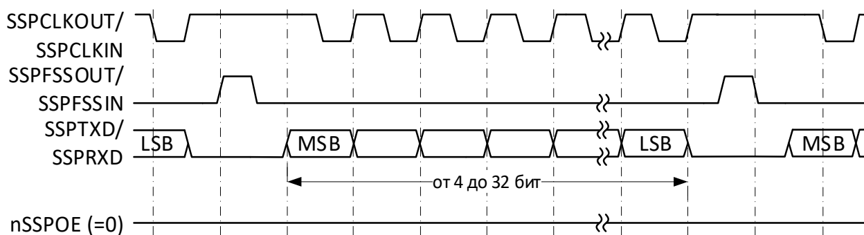
Рисунок 86 – Формат синхронного обмена протокола SPI, SPO=1, SPH=0 (непрерывный обмен)
