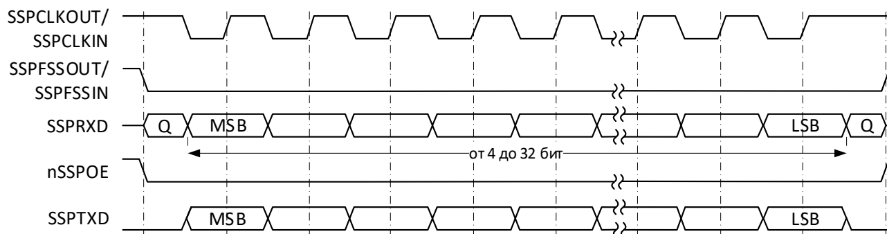
Рисунок 87 – Формат синхронного обмена протокола SPI, SPO=1, SPH=1
