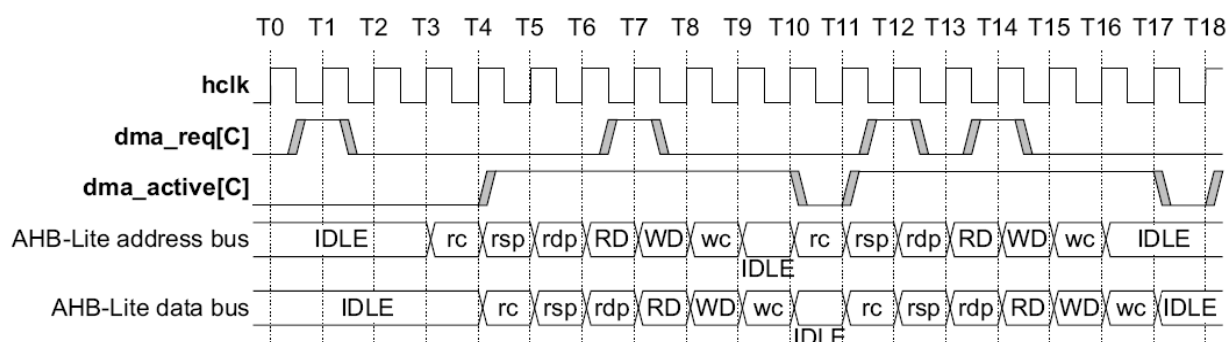
Рисунок 103 – Диаграмма работы при получении импульсного запроса от периферийного блока
