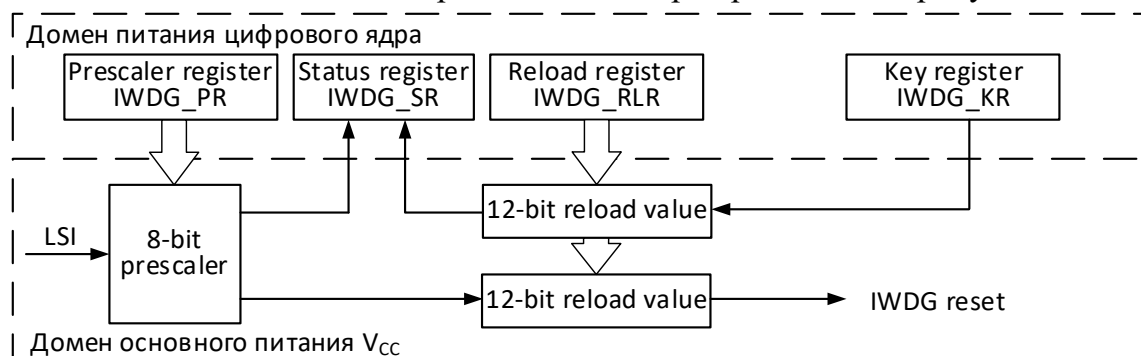
Рисунок 117 – Блок-схема независимого сторожевого таймера
