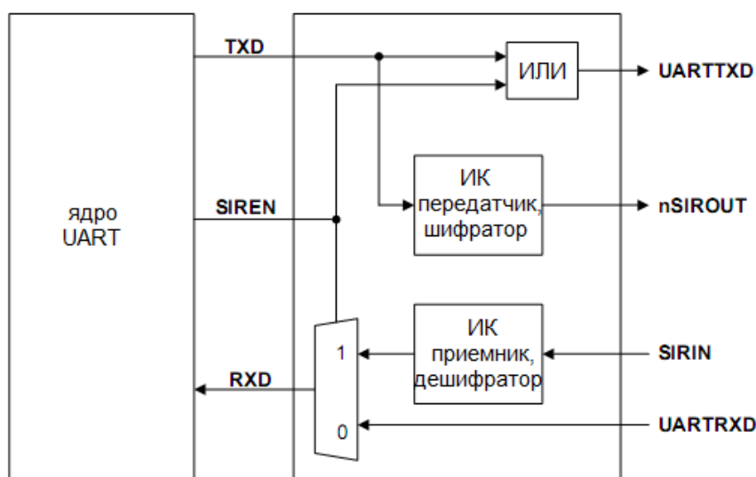
Рисунок 96 – Структурная схема кодека IrDA
