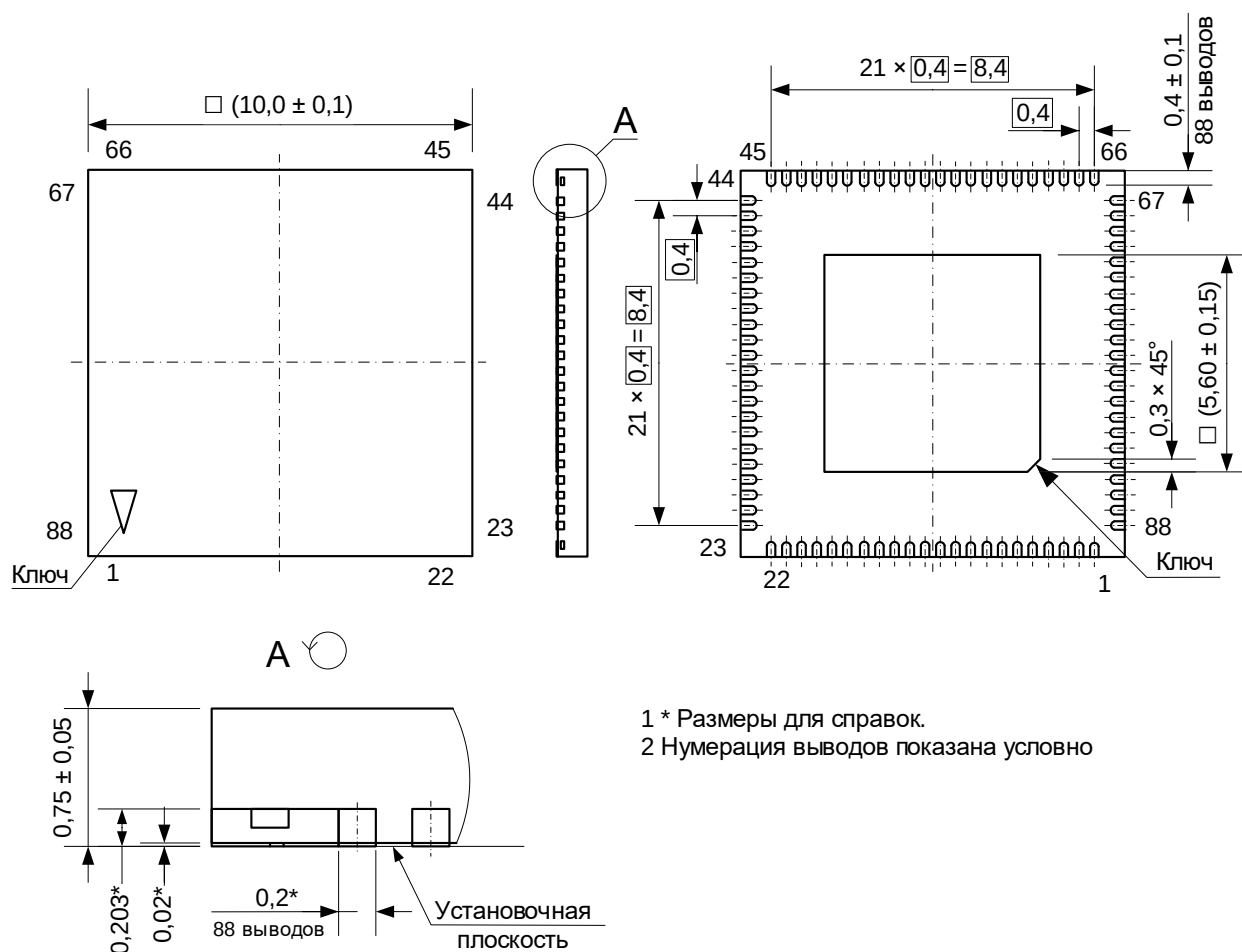
Рисунок 152 – Микросхемы MDR1206FI, MDR1206AFI в корпусе QFN88 10×10×0,75 (0,4)
