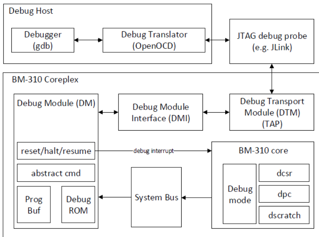
Рисунок 114 – Архитектура системы отладки
