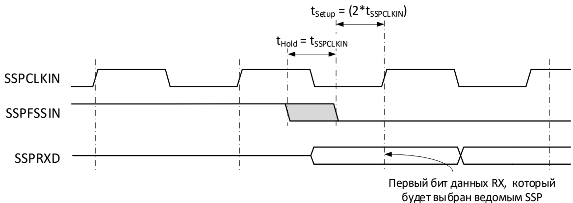
Рисунок 90 – Формат Microwire, требования к времени установки и удержания сигнала SSPFSSIN
