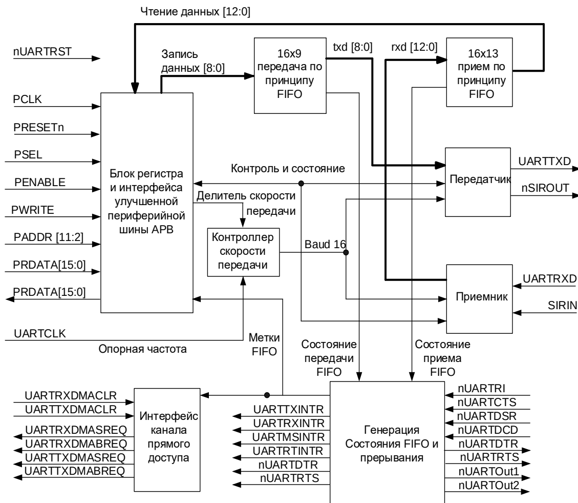
Рисунок 95 – Блок-схема универсального асинхронного приёмопередатчика (UART)
