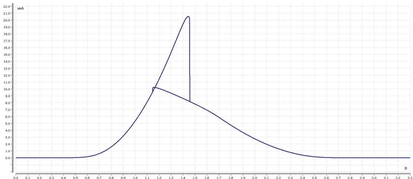
Рисунок 144 – Типовая зависимость дополнительного тока потребления по питанию U_{CCB} от напряжения на входе WAKEUP1-WAKEUP3 при U_{CCB} = 3.3 В в НУ
