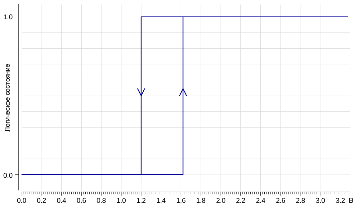
Рисунок 145 – Типовая зависимость логического состояния от напряжения на цифровом входе порта ввода-вывода при U_{CC} = 3,3 В в НУ
