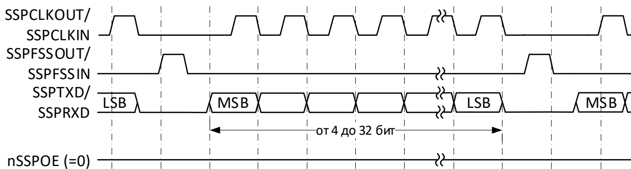
Рисунок 83 – Формат синхронного обмена протокола SPI, SPO=0, SPH=0 (непрерывный обмен)
