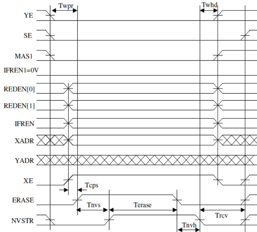
Рисунок 18 – Временная диаграмма стирания страницы памяти
