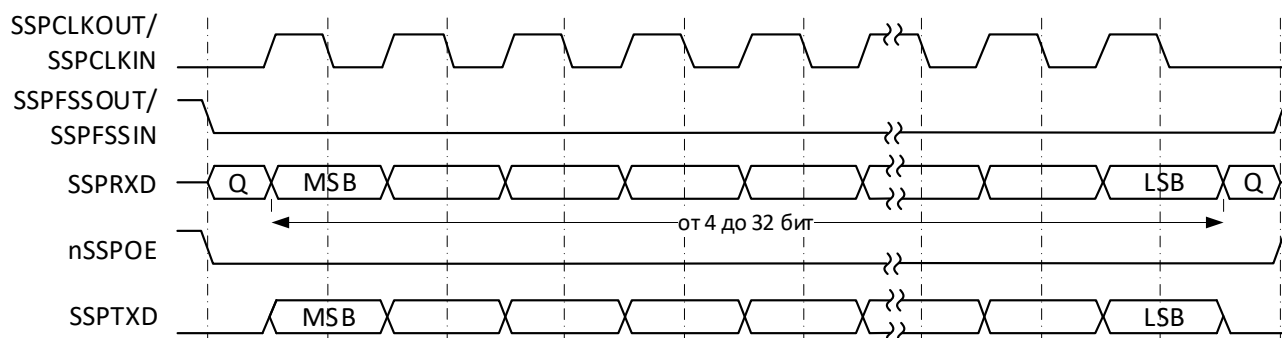
Рисунок 84 – Формат синхронного обмена протокола SPI, SPO=0, SPH=1
