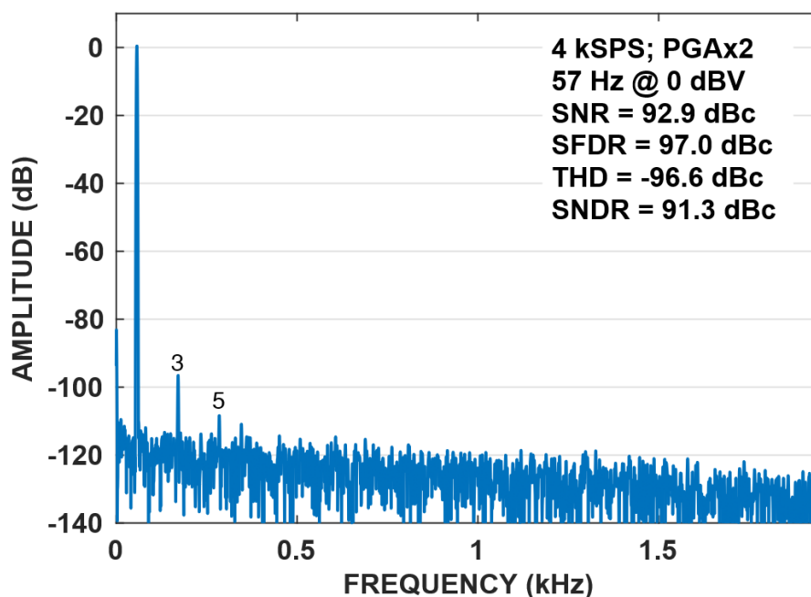
Рисунок 141 – Типовой спектр в НУ для \Delta\Sigma АЦП микросхем MDR1206AFI (CHIP_ID = 215) в канале F2IDAT для дифференциального входного сигнала +/- 1 В (0.707 RMS). Усиление = 6 дБ (F2IGAIN = 00)
