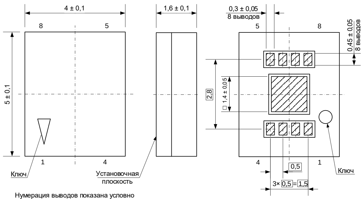
Рисунок 153 – Микросхемы MDR1215LGI в корпусе LGA8 4×5×1,6 (0,5)
