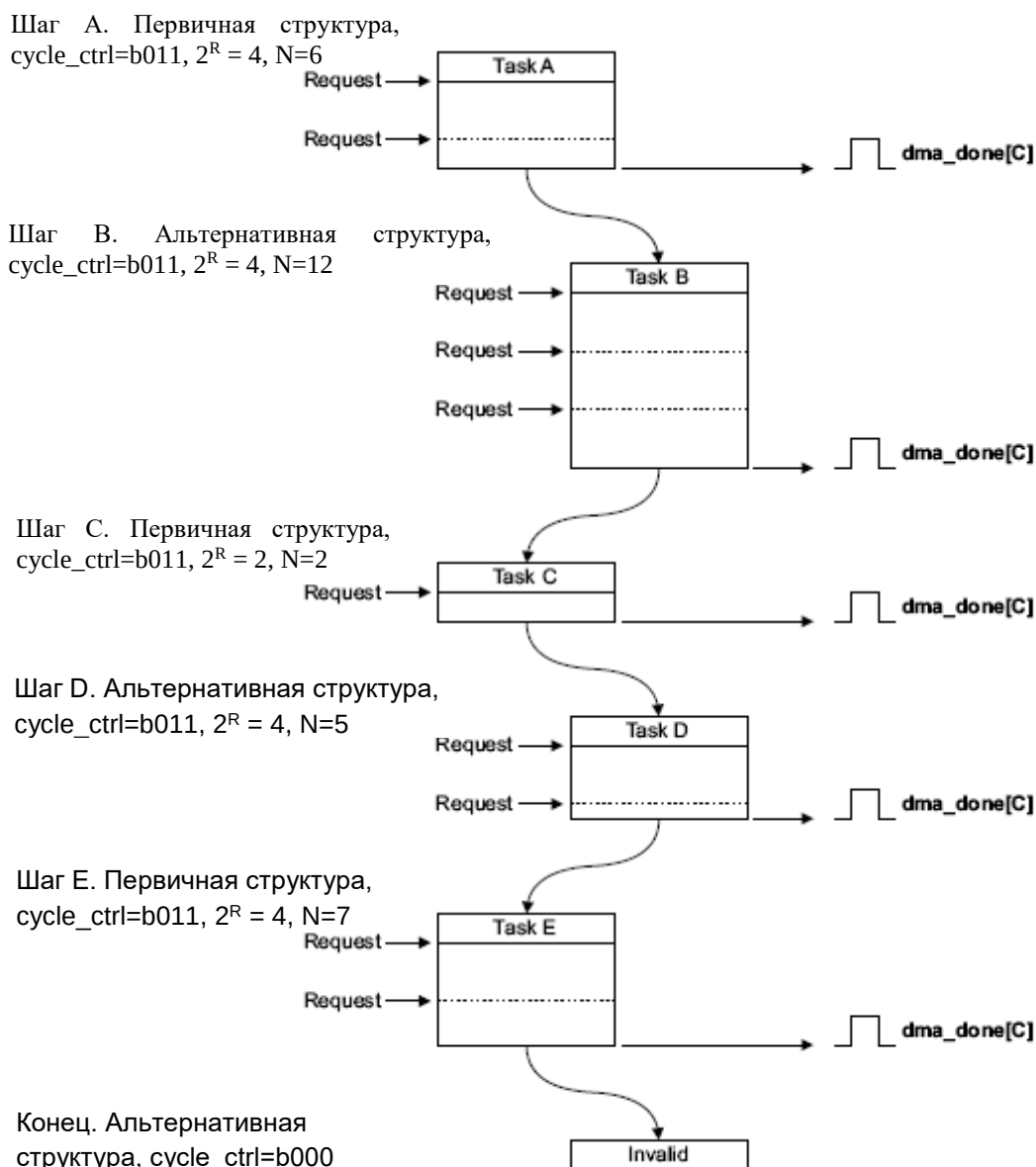
Рисунок 109 – Пример функционирования контроллера в режиме «пинг-понг»
