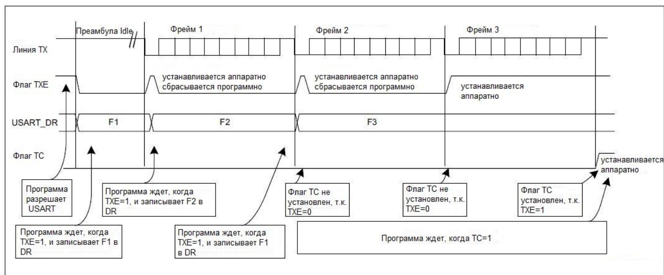
Рисунок 124 – Состояние TC/TXE во время передачи
