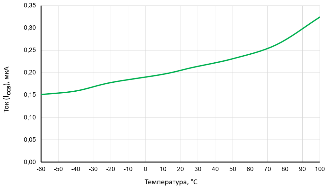
Рисунок 148 – Зависимость статического тока потребления I_{CCB} батарейного домена микросхем MDR1206FI (CHIP_ID = 217) от температуры при U_{CCB} = 3,3 В
