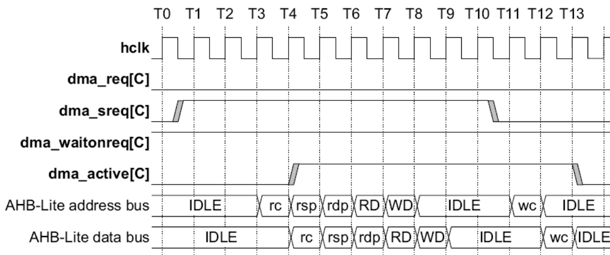
Рисунок 107 – Работа DMA при использовании dma_waitonreq совместно с dma_sreq
