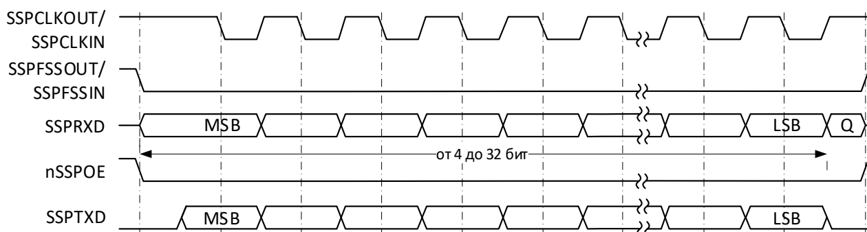
Рисунок 85 – Формат синхронного обмена протокола SPI, SPO=1, SPH=0 (одиначный обмен)
