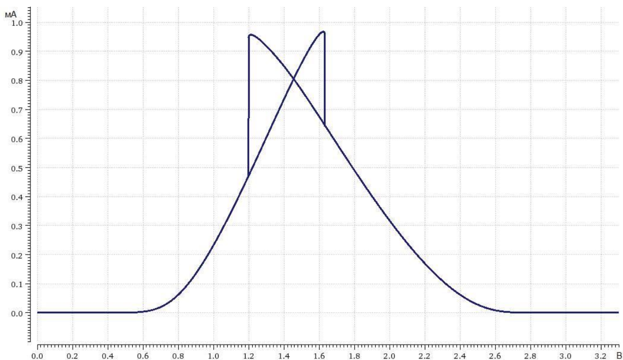
Рисунок 143 – Типовая зависимость дополнительного тока потребления по питанию U_{CC} от напряжения на цифровом входе порта ввода-вывода при U_{CC} = 3.3 В в НУ
