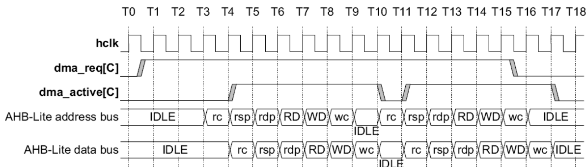
Рисунок 104 – Диаграмма работы при получении запроса на обработку по уровню
