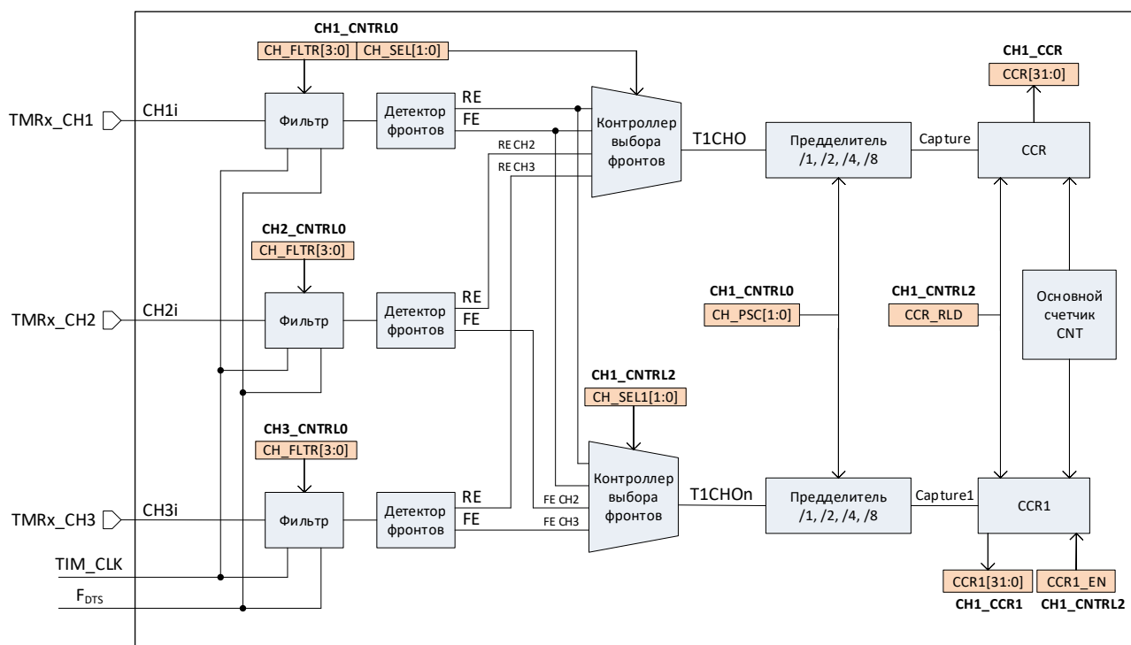
Рисунок 61 – Структурная схема блока захвата на примере канала 1
