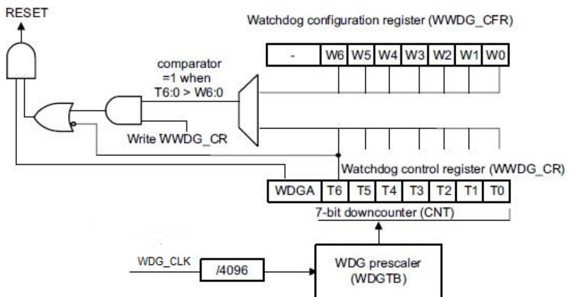
Рисунок 118 – Блок-схема оконного сторожевого таймера
