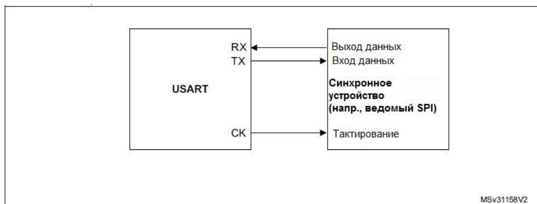
Рисунок 130 – Пример синхронной передачи USART
