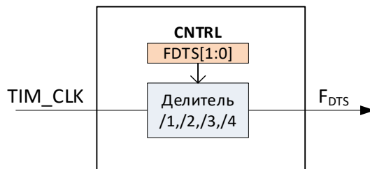
Рисунок 50 – Схема формирования тактовой частоты F DTS
