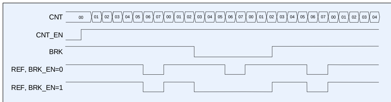
Рисунок 67 – Диаграмма сброса сигнала REF по выводу BRK
