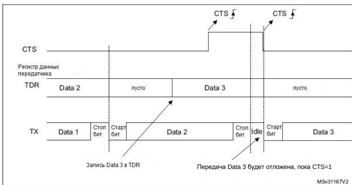
Рисунок 138 – Управление потоком CTS
