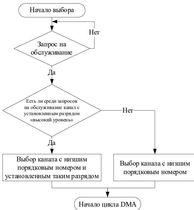
Рисунок 108 – Алгоритм выбора следующего канала для обслуживания
