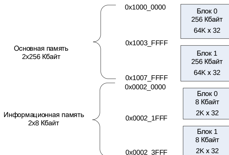
Рисунок 16 – Структура памяти
