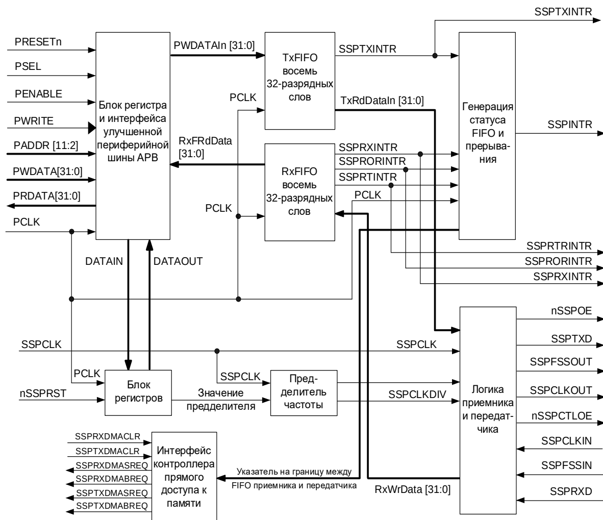
Рисунок 79 – Структурная схема модуля SSP
