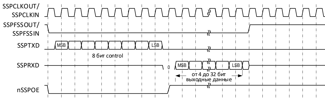
Рисунок 88 – Формат синхронного обмена протокола Microwire (одиночный обмен)
