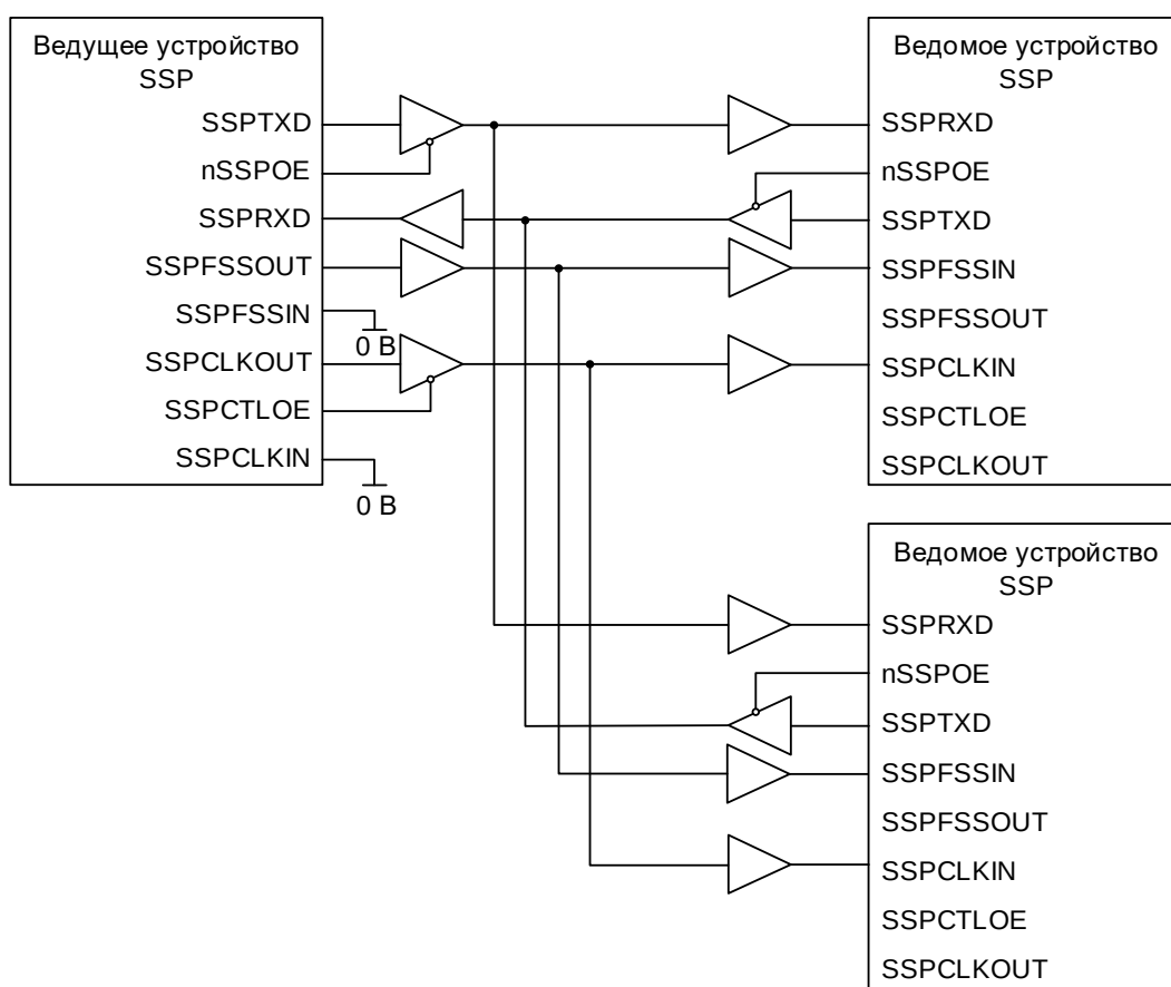
Рисунок 91 – Ведущее устройство SSP подключено к двум ведомым
