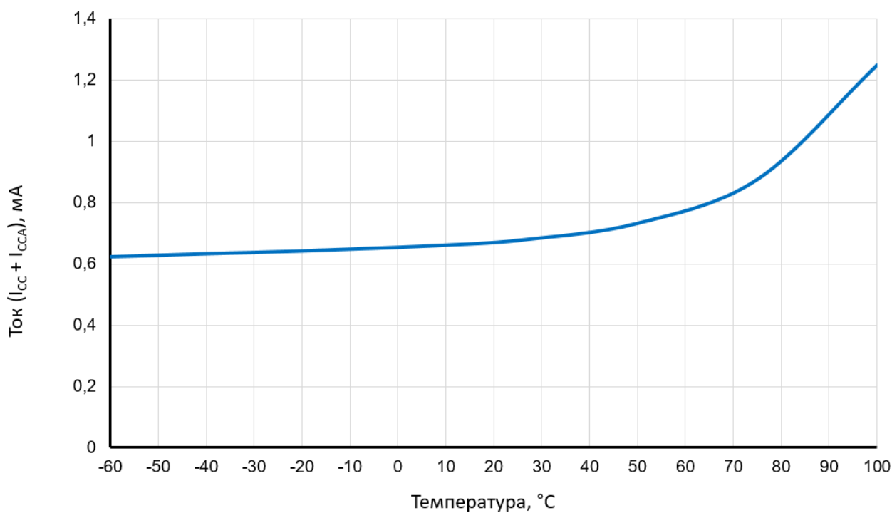
Рисунок 150 – Зависимость суммарного статического тока ( nRESET = 0 ) I_{CC} и I_{CCA} микросхем MDR1206FI (CHIP_ID = 217) от температуры при U_{CC} = U_{CCA} = 3,3 В
