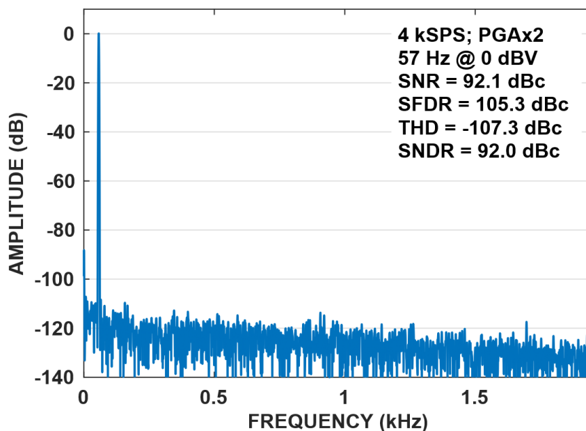
Рисунок 140 – Типовой спектр в НУ для \Delta\Sigma АЦП микросхем MDR1206FI (CHIP_ID = 217) в канале F2IDAT для дифференциального входного сигнала +/- 1 В (0.707 RMS). Усиление = 6 дБ (F2IGAIN = 00)
