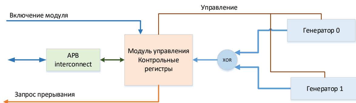
Рисунок 120 – Структурная схема блока генератора случайных чисел
