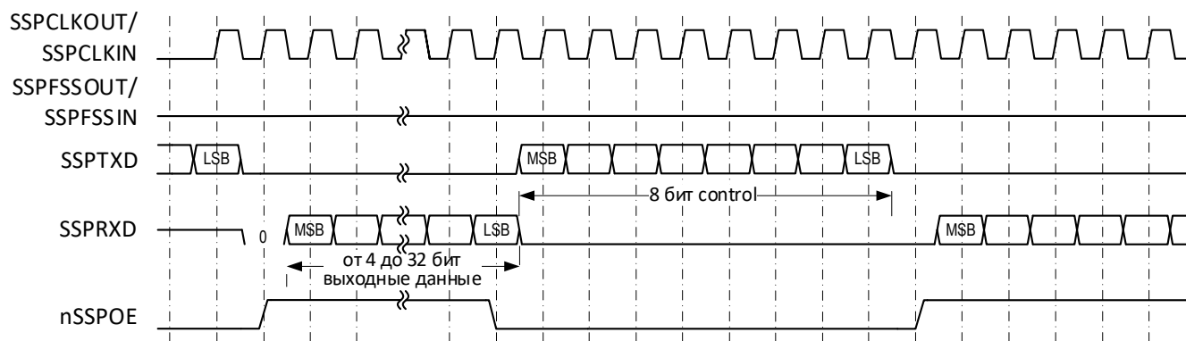
Рисунок 89 – Формат синхронного обмена протокола Microwire (непрерывный обмен)
