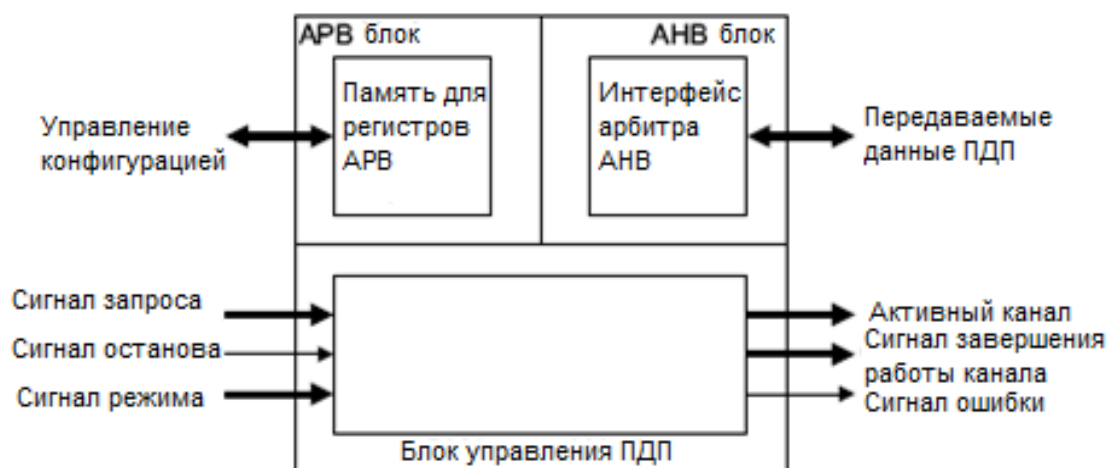
Рисунок 102 – Структурная схема контроллера
