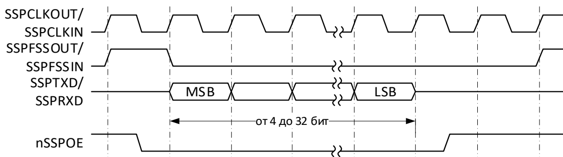
Рисунок 80 – Формат синхронного обмена протокола SSI (единичный обмен)
