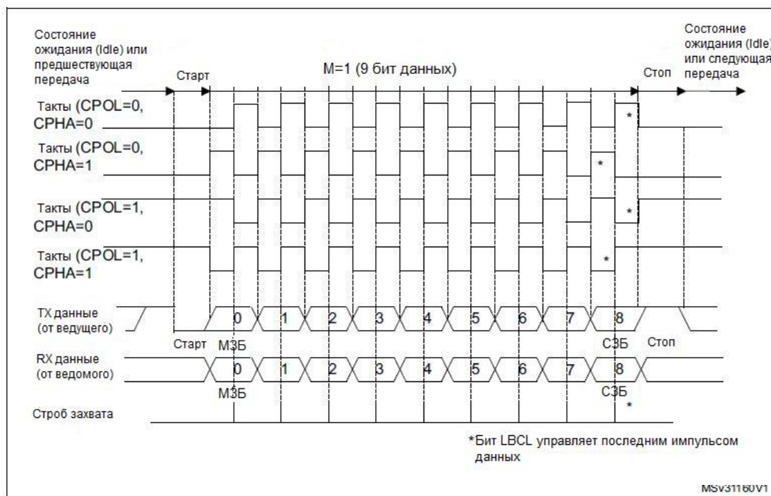
Рисунок 132 – Диаграмма тактирования данных USART (M=1)
