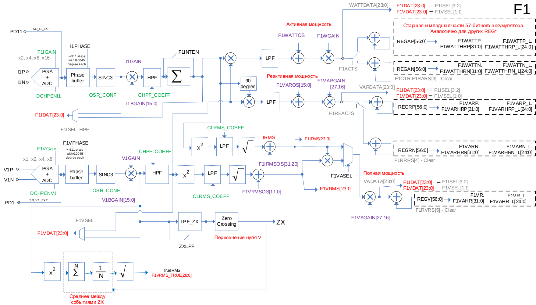
Рисунок 28 – Структурная схема F1
