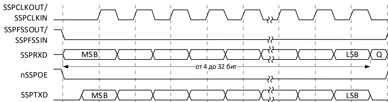
Рисунок 82 – Формат синхронного обмена протокола SPI, SPO=0, SPH=0 (одиночный обмен)
