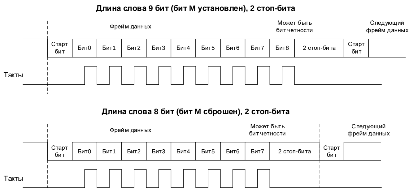
Рисунок 122 – Программирование длины слова
