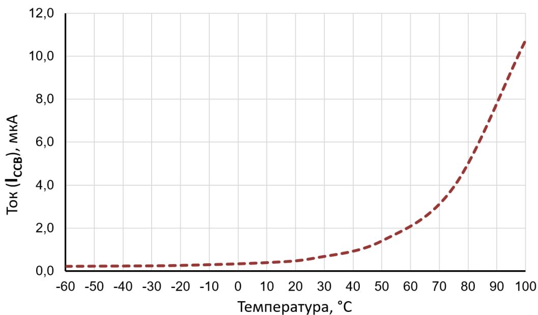
Рисунок 149 – Зависимость статического тока потребления I_{CCB} батарейного домена микросхем MDR1206FI (CHIP_ID = 217) от температуры при U_{CCB} = 3,3 В и отсутствии основного питания
