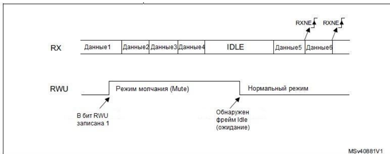
Рисунок 128 – Режим молчания (Mute) с обнаружением линии Idle
