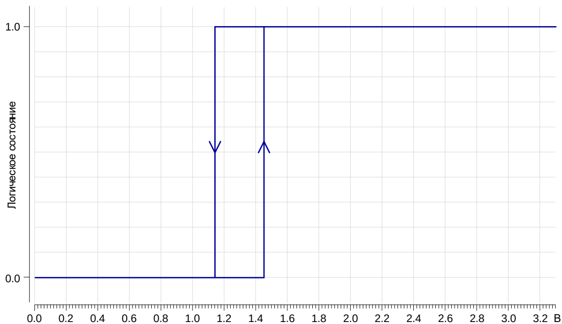
Рисунок 146 – Типовая зависимость логического состояния от напряжения на входе WAKEUP1-WAKEUP3 при U_{CCB} = 3,3 В в НУ
