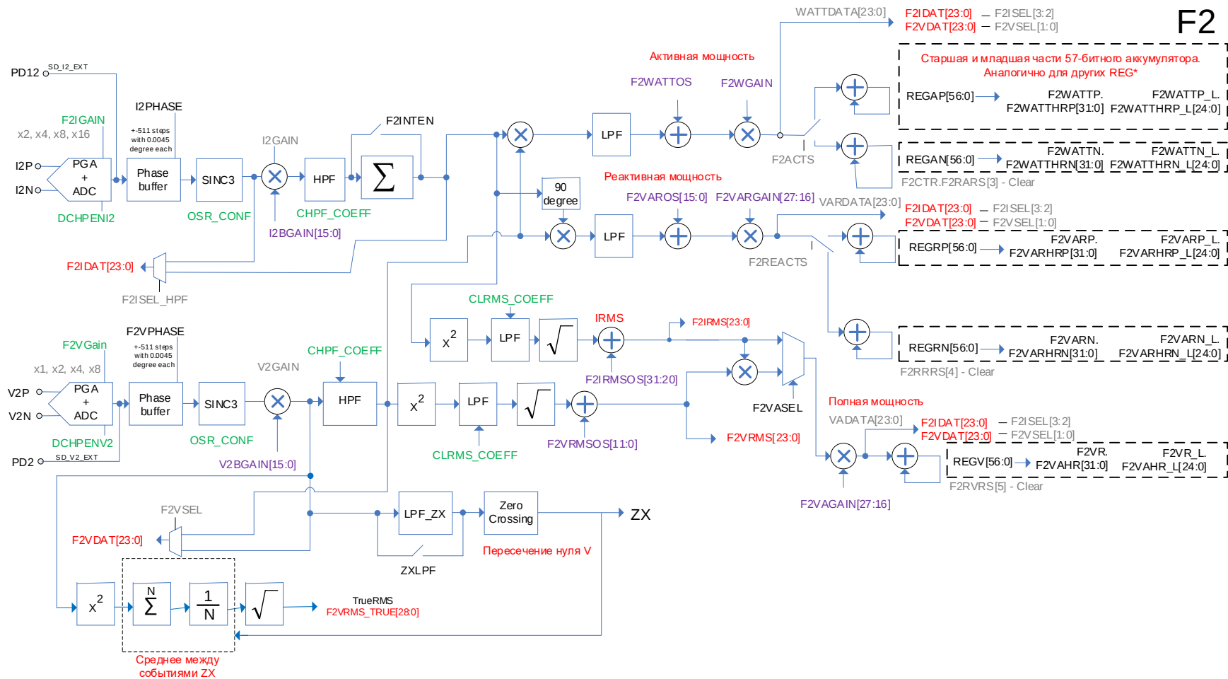
Рисунок 29 – Структурная схема F2
