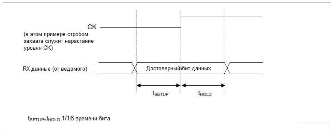
Рисунок 133 – Время установки/удержания RX
