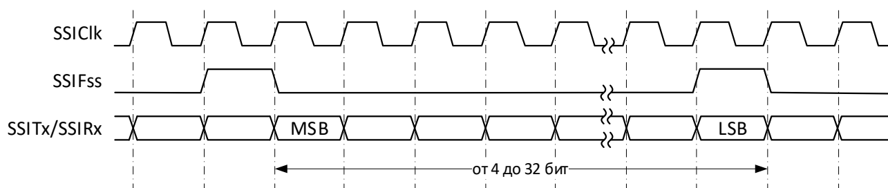
Рисунок 81 – Формат синхронного обмена протокола SSI (непрерывный обмен)
