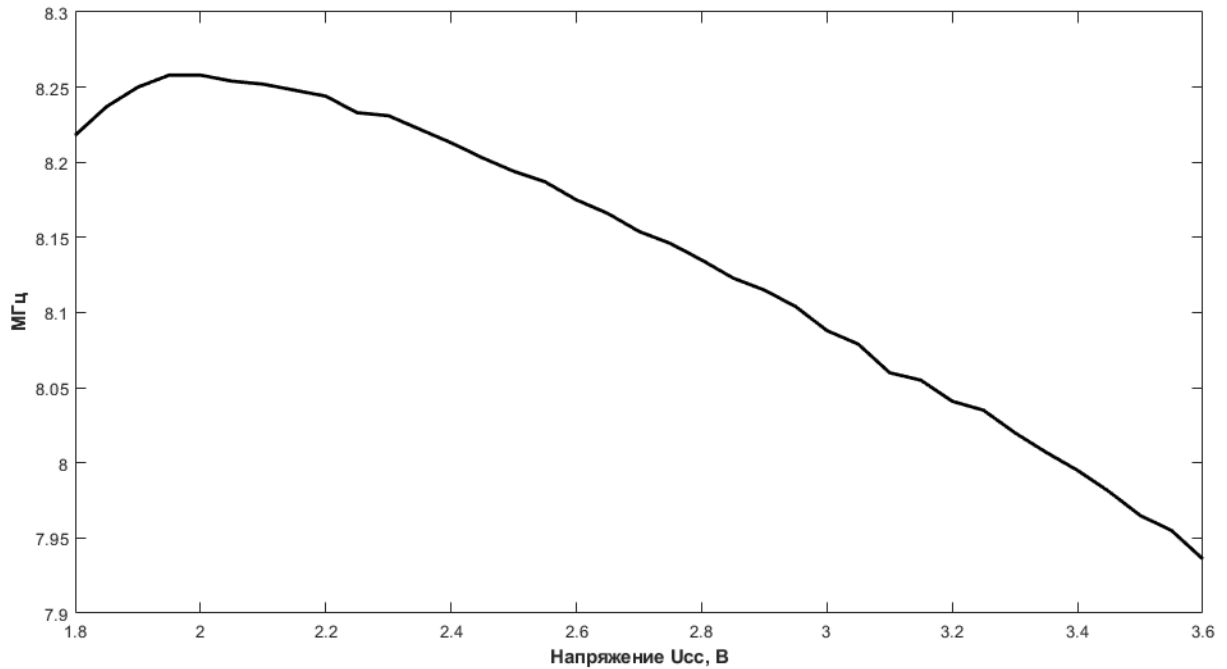
Рисунок 147 – Зависимость частоты RC генератора HSI микросхем MDR1206FI, MDR1215LGI (CHIP_ID = 217) от напряжения питания U_{CC} в НУ
