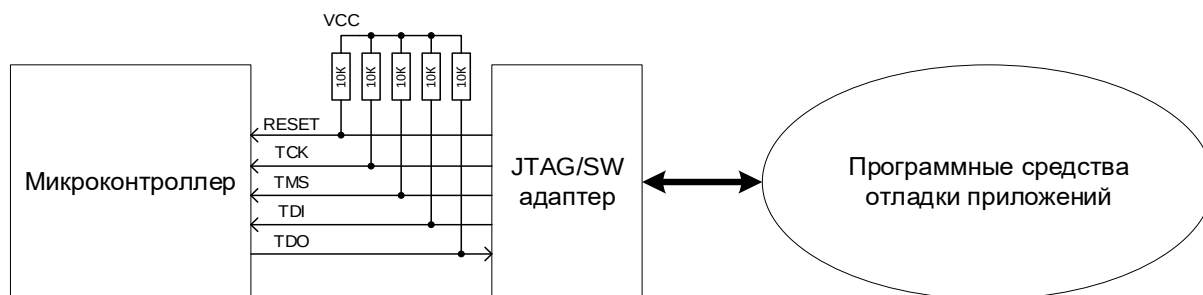
Рисунок 116 – Схема работы в режиме отладки
