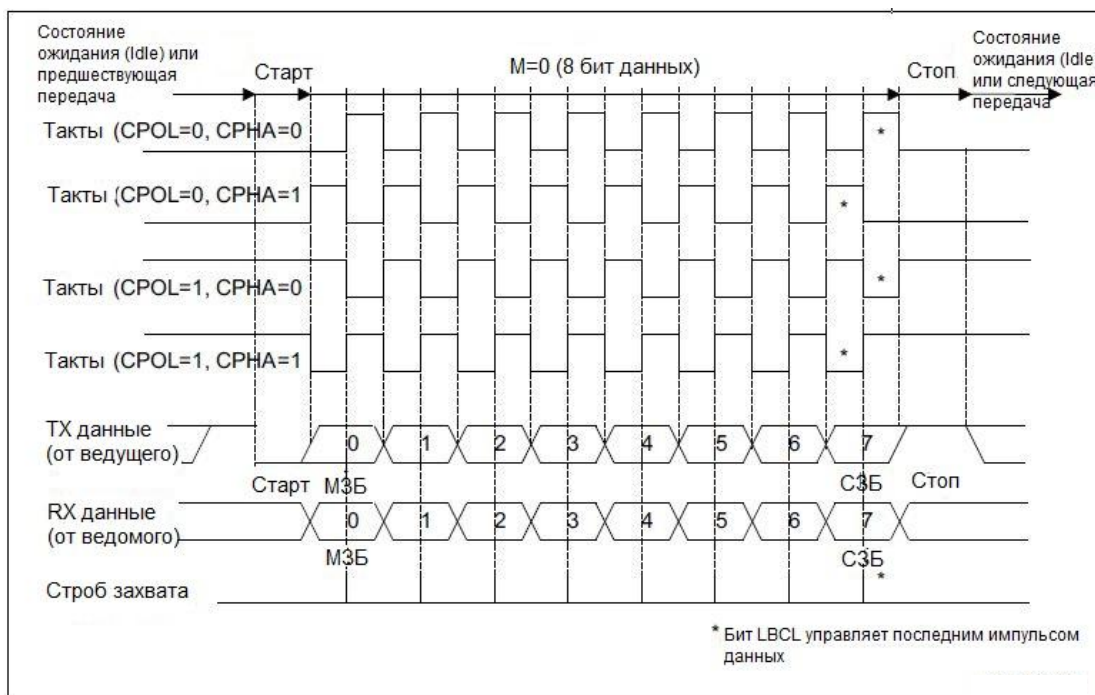
Рисунок 131 – Диаграмма тактирования данных USART (M=0)
