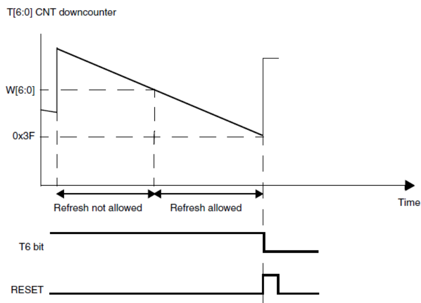
Рисунок 119 – Временная диаграмма оконного сторожевого таймера
