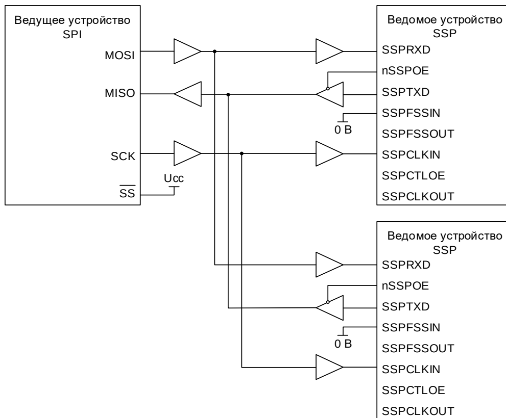
Рисунок 93 – Ведущее устройство, протокол SPI, подключено к двум ведомым модулям SSP
