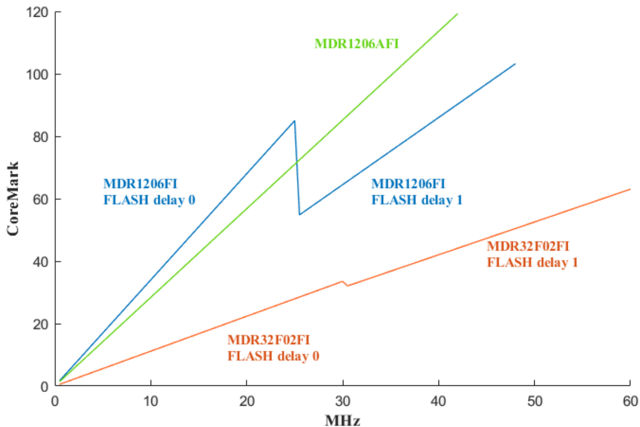
Рисунок 142 – Производительность в Coremark при выполнении из Flash-памяти
